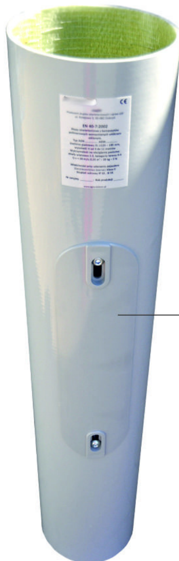
Drzwiczki rewizyjne (PC + ABS)
