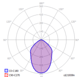
EMLB 2 Ex z odbłyśnikiem symetrycznym
