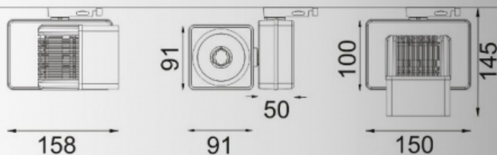
LED 39W 16°
