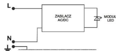
Rys. 2. Ideowy schemat podłączenia elektrycznego oprawy M40A wyposażonej w źródło światła LED Fig. 2 Luminaire M40A LED electrical connection diagram
