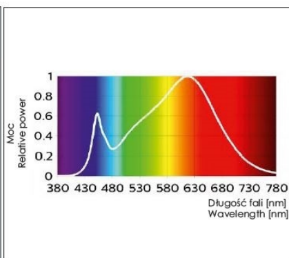
Rys. 4 Rozkład widmowy oprawy M40A (30W LED) Fig. 4 Spectral distribution of M40A (30W LED) luminaire
