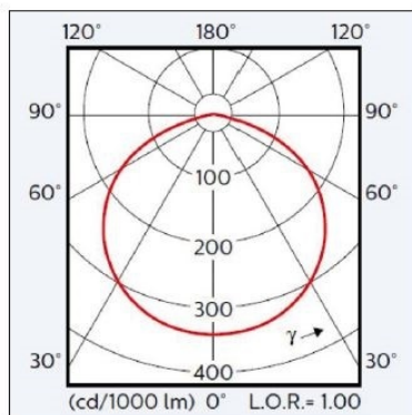
Rys. 3 Wykres światłości oprawy M40A Fig. 3 Luminaire M40A light graph.
